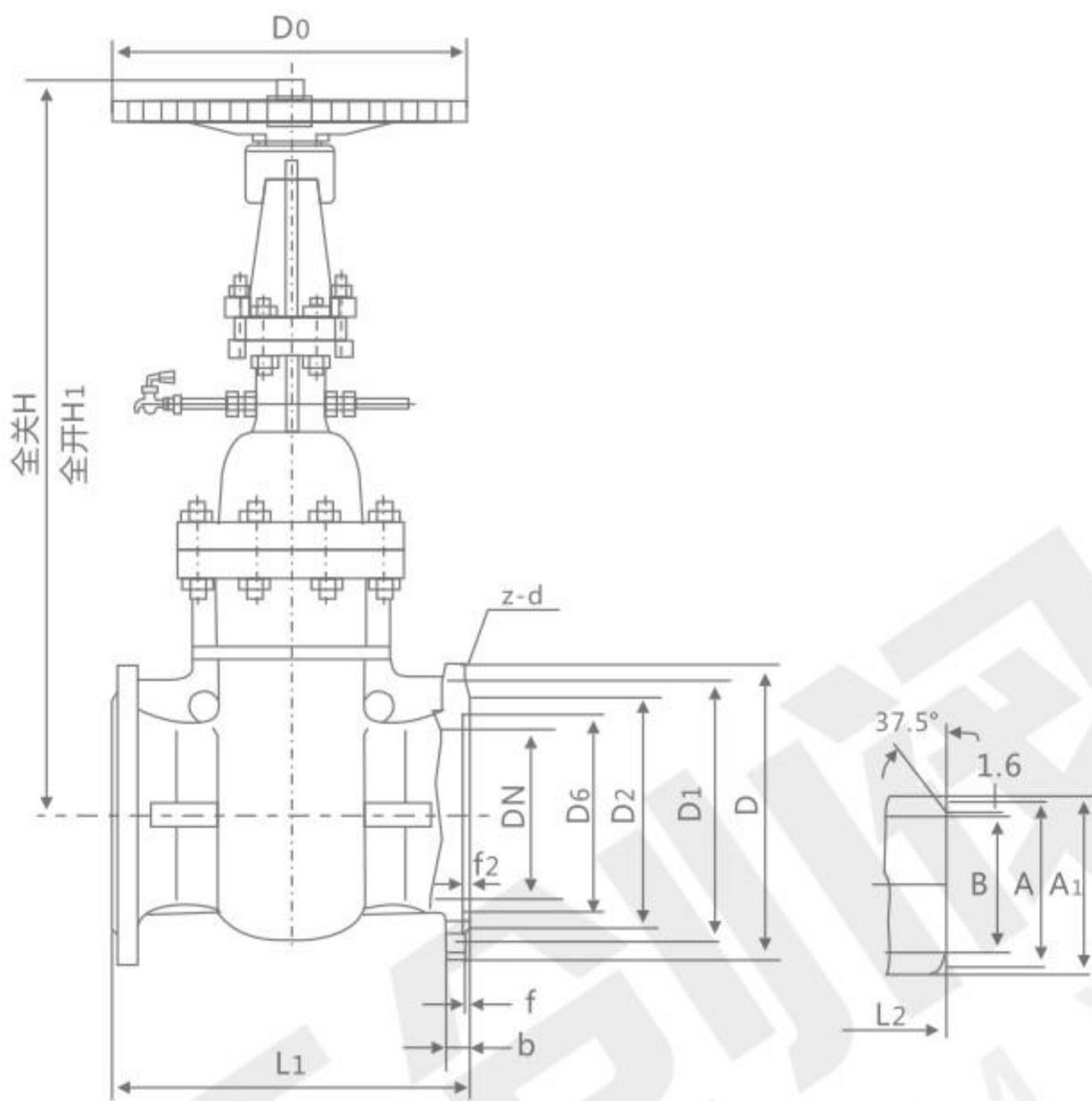
主要外形尺寸及重量Main dimensions and weight JB/T79.2-1994
